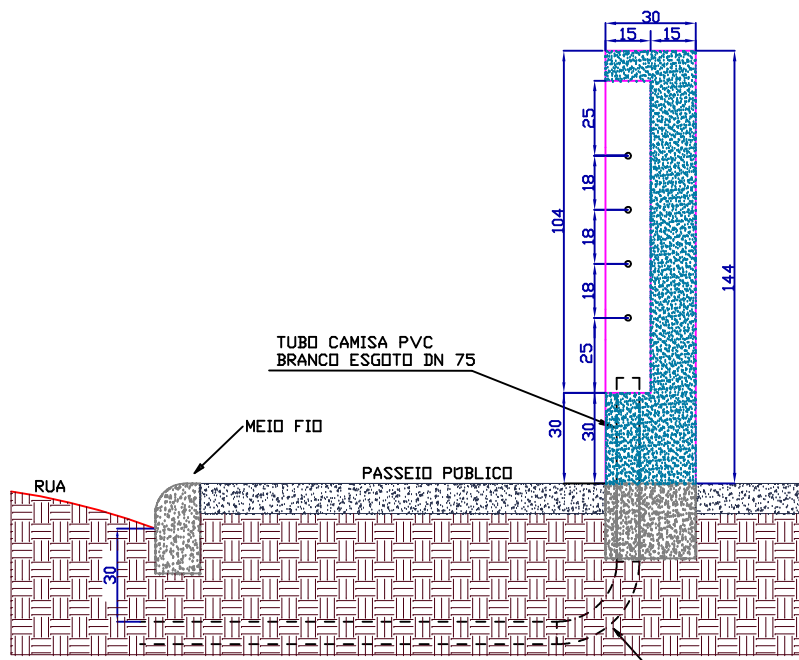
CORTE TRANSVERSAL
